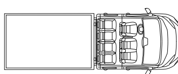
Pritschenwagen mit Doppelkabine L4
