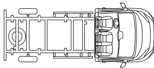
Leiterrahmen L3
